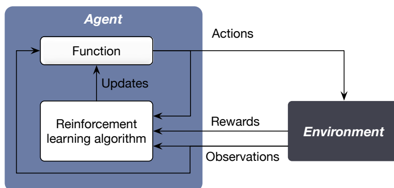
图 2-10 强化学习。
