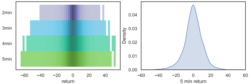
图 4-2 上证 50 指数收益率分布。左图为 2、3、4、5 分钟收益率分布的比较，右图为 5 分钟收益率分布曲线。
